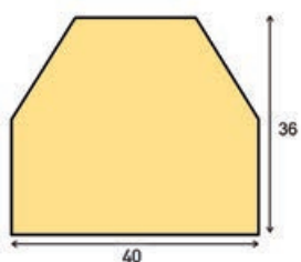
Flächenschutz Trapez, Typ CC
