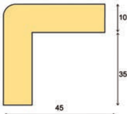
Kantenschutz Winkel, Typ H
